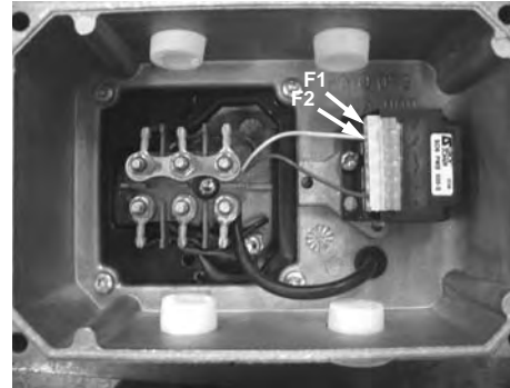
F1 and F2 terminals of the VMA ESFR 31/32 option
